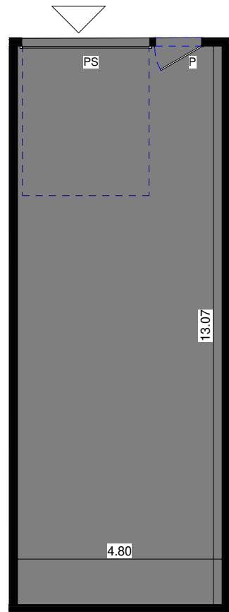
PLAN RDC
