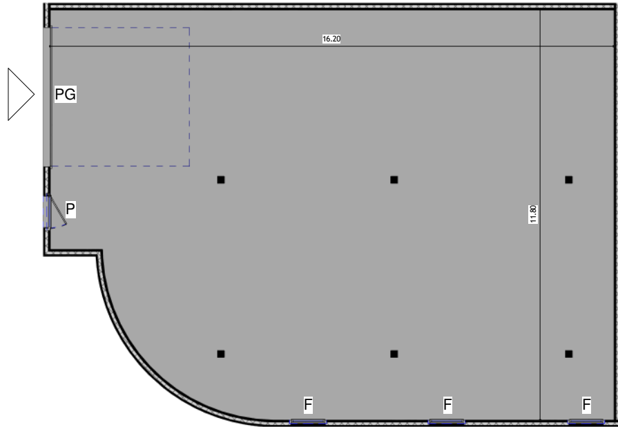
PLAN RDC
